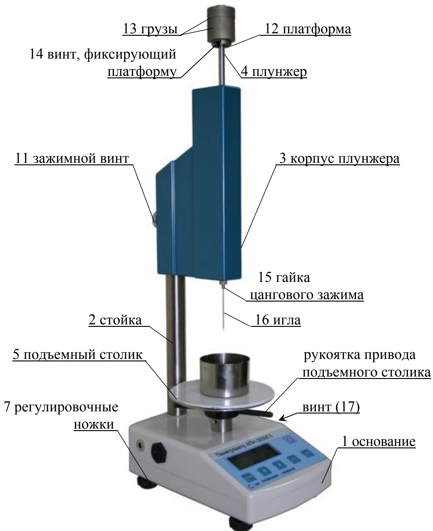
Рисунок 1 - Общий вид прибора АПН-360МГ4
